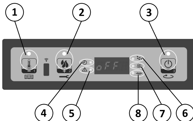
Fig. 3 - Οθόνη: led αναμμένα
