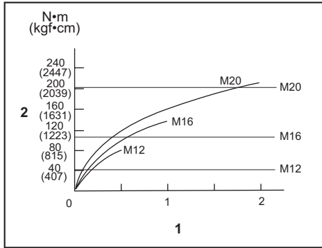
1. Tiempo de apriete (segundo) 2. Par de apriete
