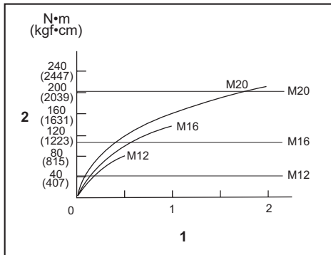
1. Tempo de aperto (segundos) 2. Binário de aperto
