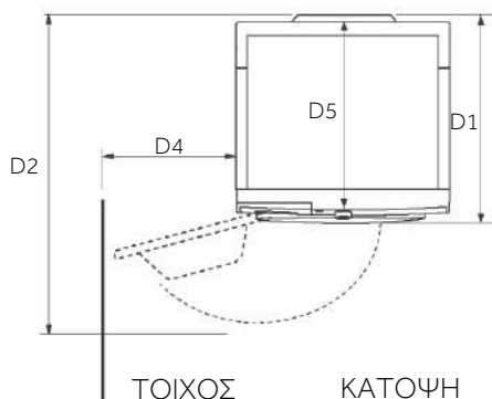
ΤΟΙΧΟΣ
