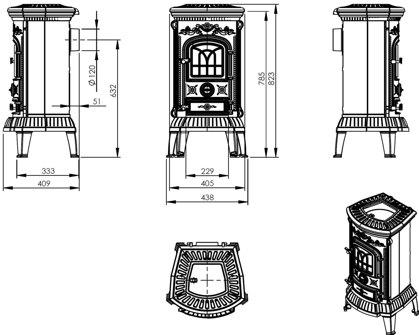
Rys. 1. [PL] Wymiary gabarytowe/ [CZ] Rozměry/ [HU] Befoglaló méretek/ [SK] Objemové rozmery/ [EN] Overall dimensions/ [LT] Gabaritiniai matmenys/ [LV] Vispārējie izmēri/ [RU] Габаритные размеры/ [EE] Üldmõõtmed/ [GR] Συνολικές διαστάσεις/ [RO] Dimensiuni gabarit/ [BG] Габаритни размери/ [UA] Габаритні розміри/ [NL] Productafmetingen/ [HR] Ukupne dimenzije/ [TR] Boyutlar/ [PT] Dimensões gerais/ [FR] Dimensions hors tout/ [ES] Dimensiones totales
